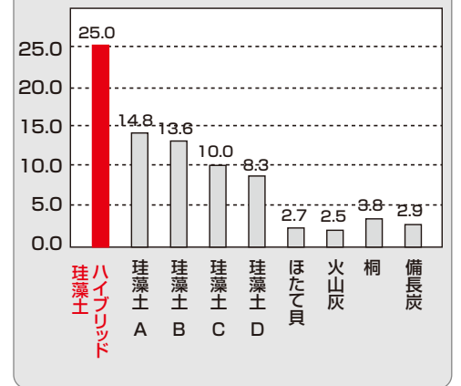
■吸放湿機能比較 【表-3】
