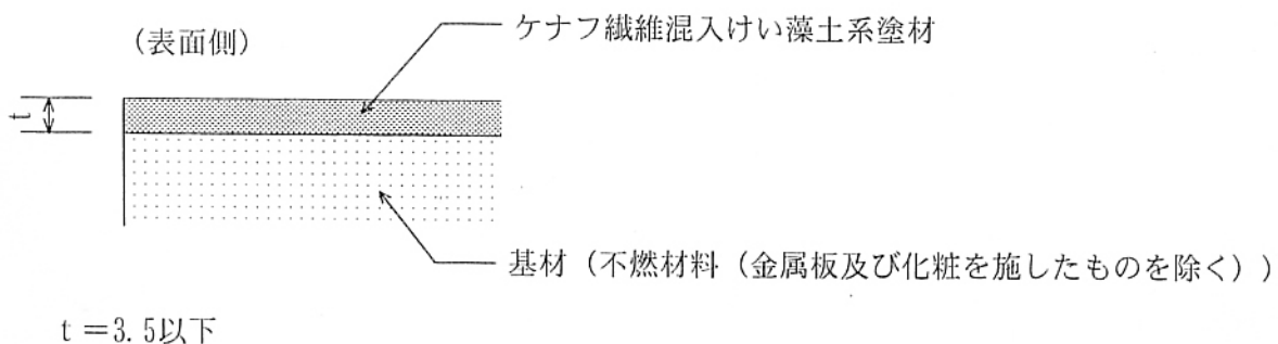
図1 断面図
